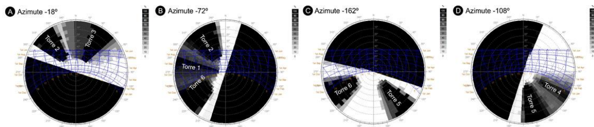
Figura 4. Sombreamento das fachadas principais.
