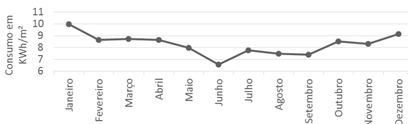
Figura 7. Consumo de energia do estudo de caso no ano de 2002.
