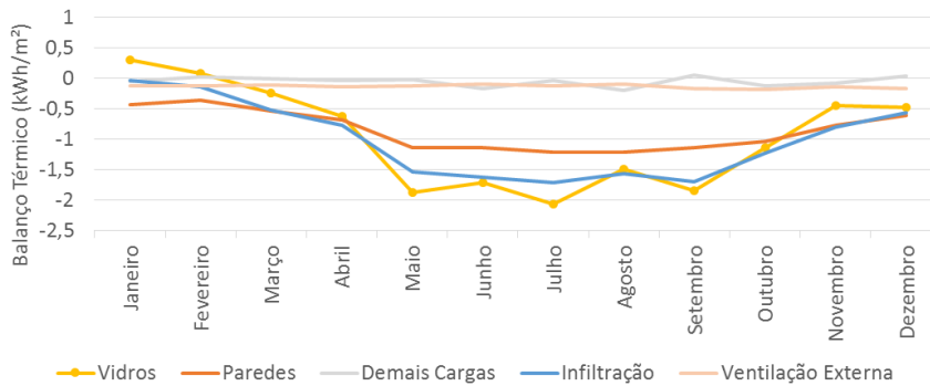
Figura 8. Balanço térmico do estudo de caso no ano de 2002.
