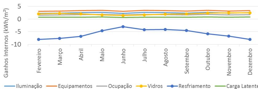
Figura 9. Ganhos internos do estudo de caso no ano de 2002.
