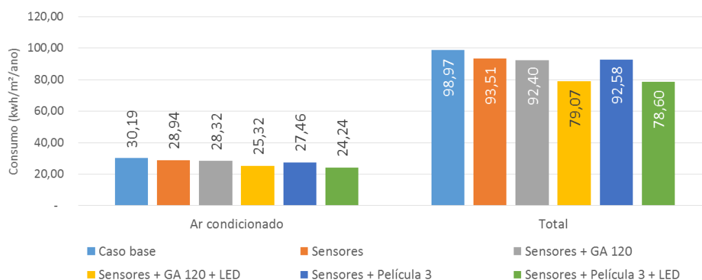
Figura 14. Consumo de energia atrelado a instalação de sensores de iluminação natural.
