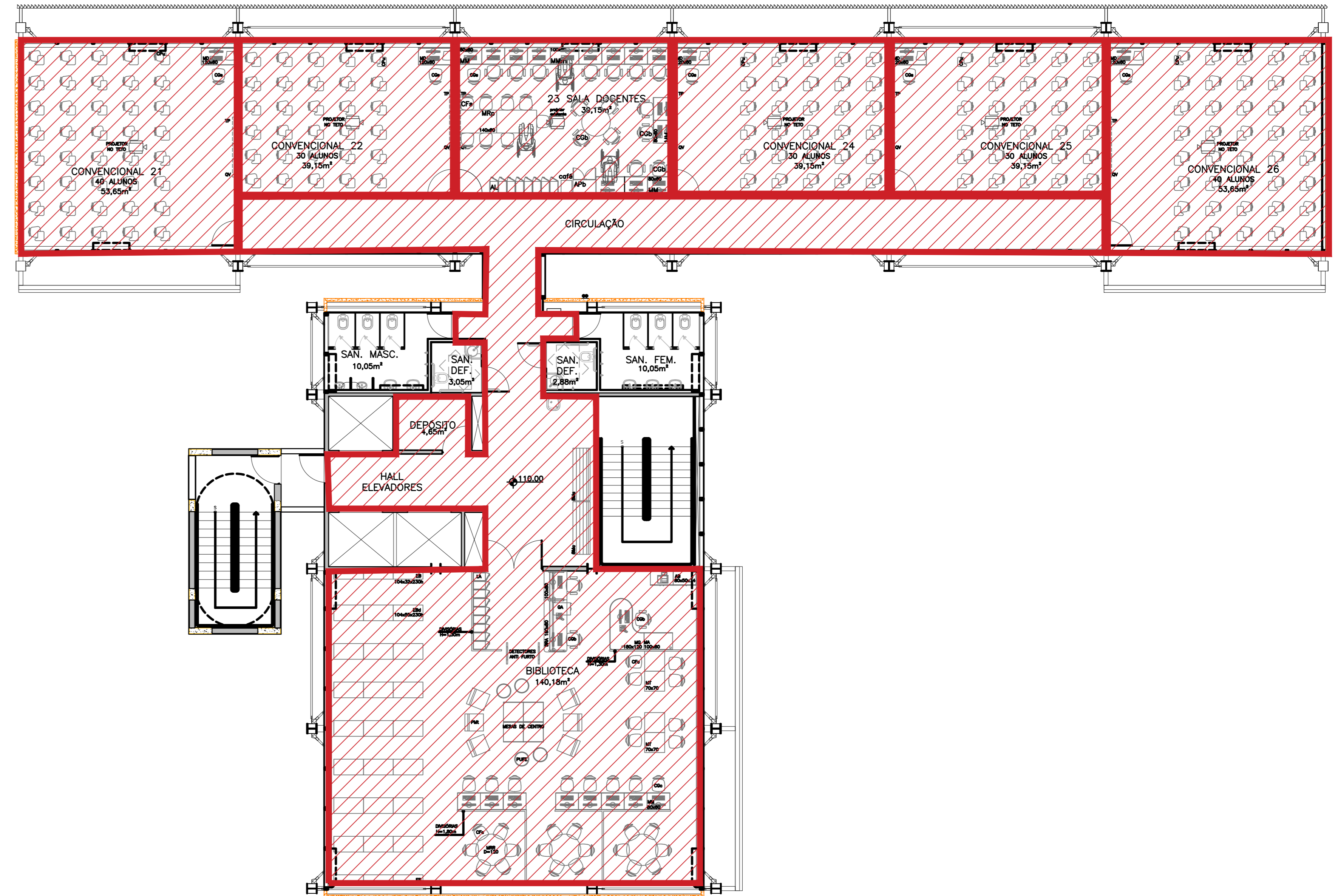
PLANTA 2º PAVIMENTO ESCALA 1:100 Área = 629,72m²
