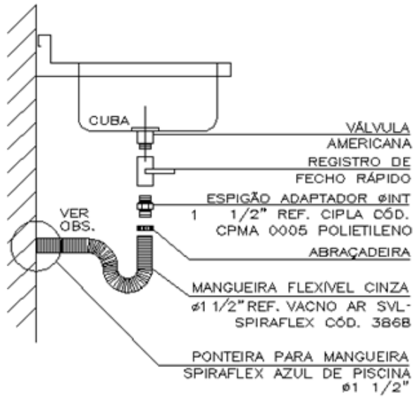
DETALHE DO SIFÃO
